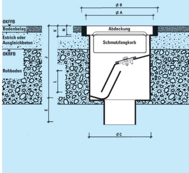
Maßangaben in mm
